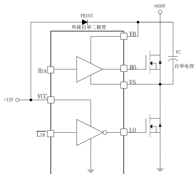
图 8-3. EG3113D 自举电路结构
